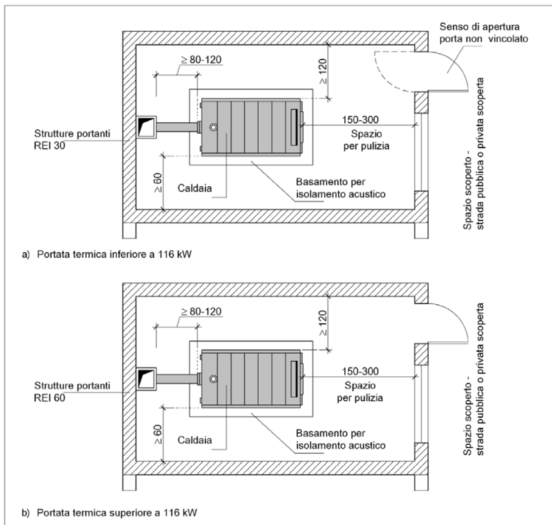
Figura 90.7 - Esempio di centrale termica alimentata a gas di rete con accesso da spazio esterno o da strada pubblica o privata scoperta. Caratteristiche costruttive e distanze minime consigliate per gli spazi attorno al generatore
