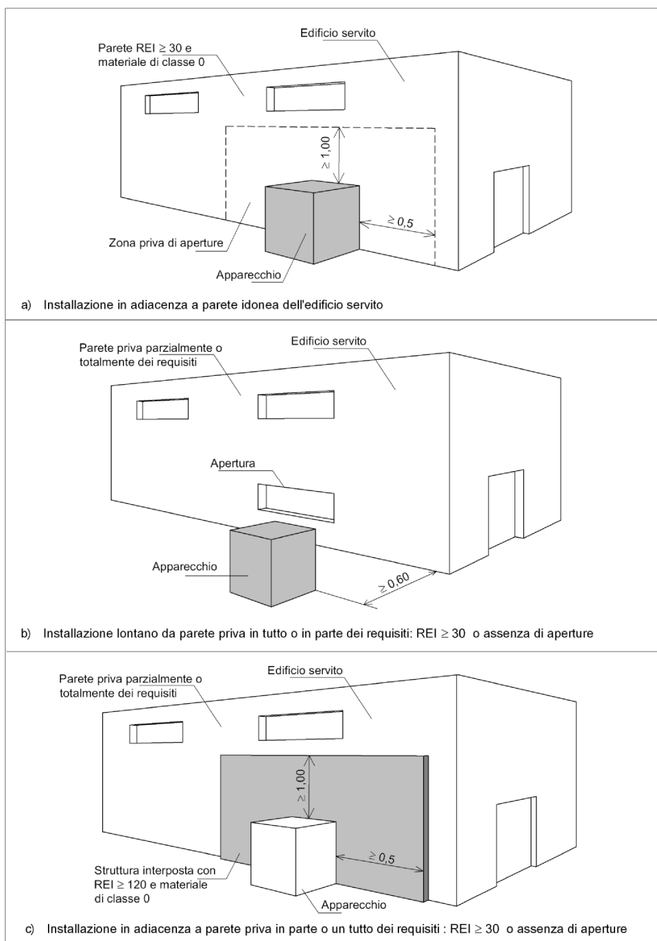
Figura 90.2 - Installazione degli apparecchi all'aperto
