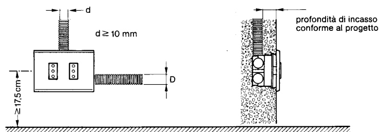
Figura 93.1 - Criteri di installazione degli impianti incassati e similari
