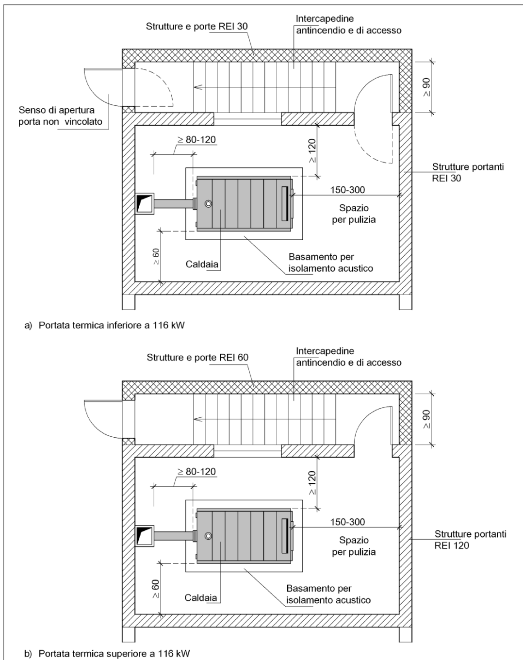
Figura 90.8 - Esempio di centrale termica alimentata a gas di rete con accesso da intercapedine antincendio di larghezza non inferiore a 0,90 m. Caratteristiche costruttive e distanze minime consigliate per gli spazi attorno al generatore
