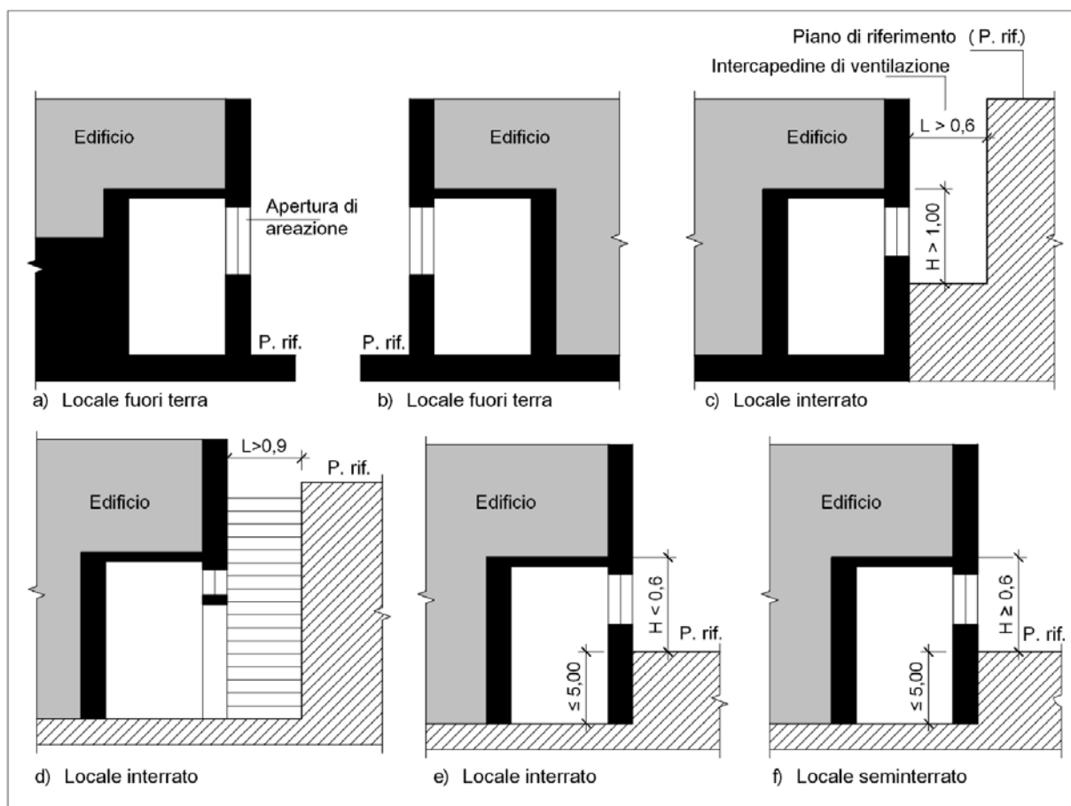
Figura 90.1 - Locali di installazione degli apparecchi degli impianti termici secondo il D.M. 12 aprile 1996
