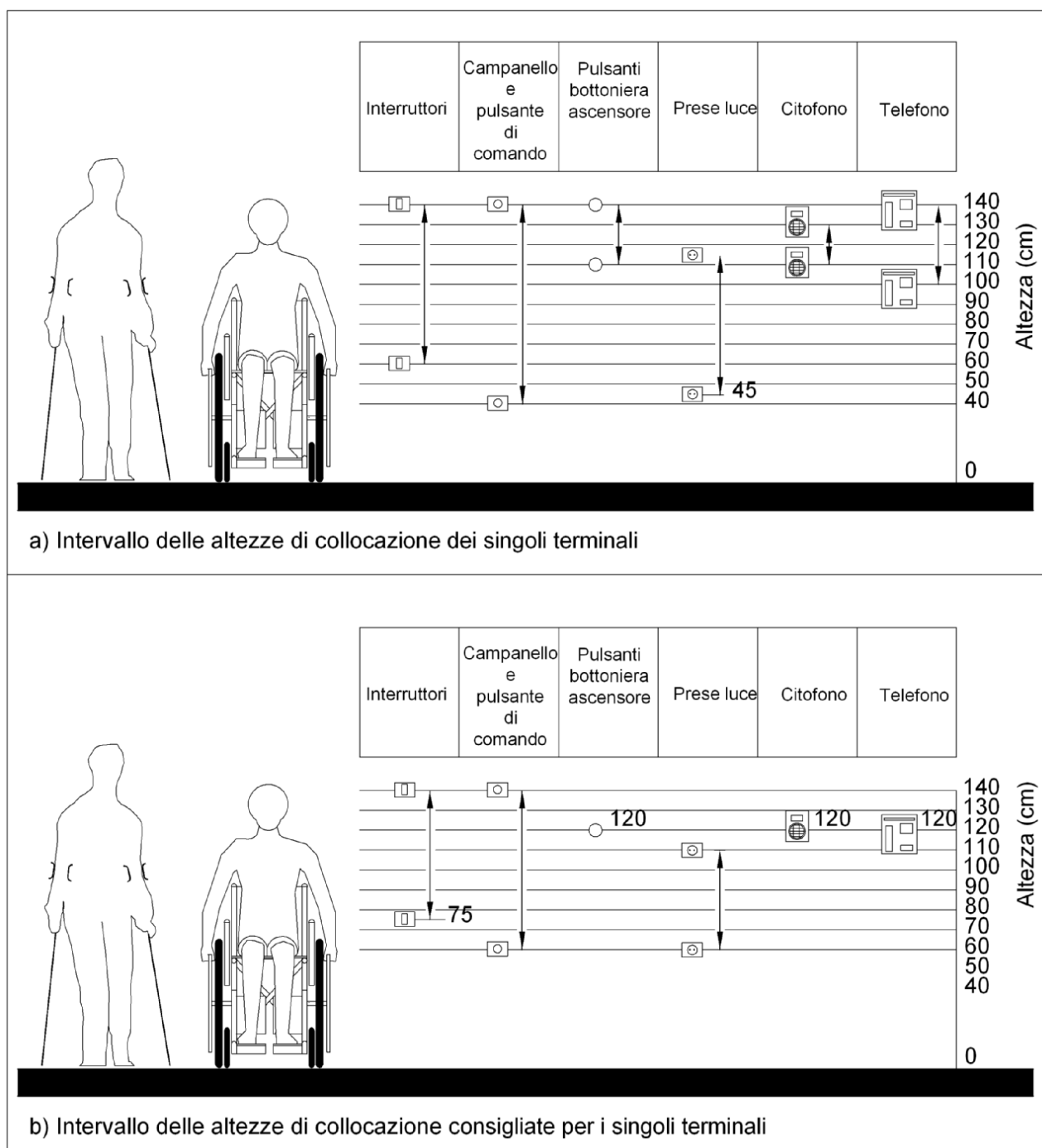
Figura 93.2 - Altezze consigliate per i terminali degli impianti elettrici e telefonici
