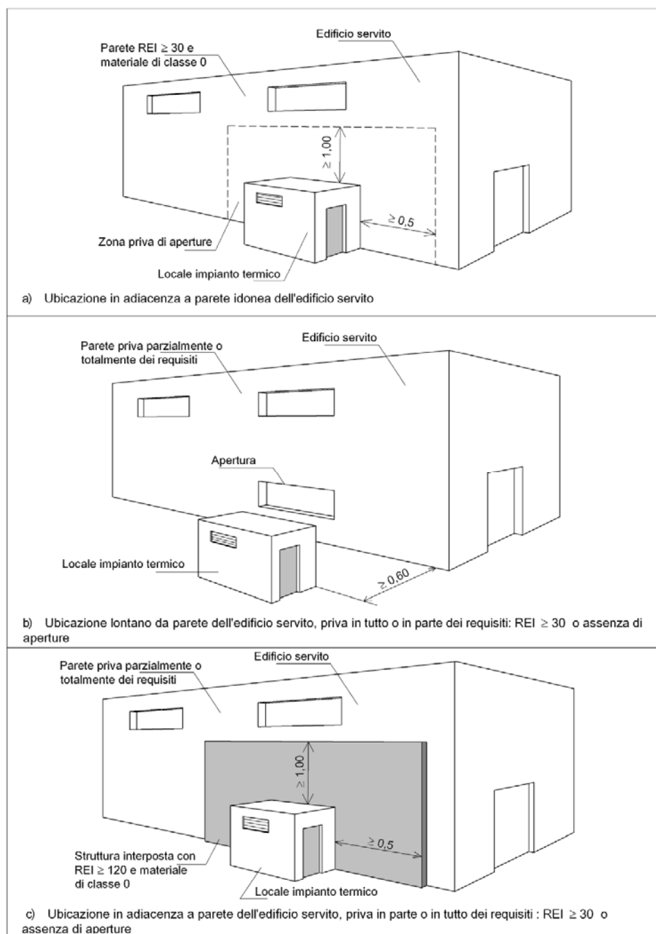
Figura 90.4 - Ubicazione dei locali esterni per l'installazione degli impianti
