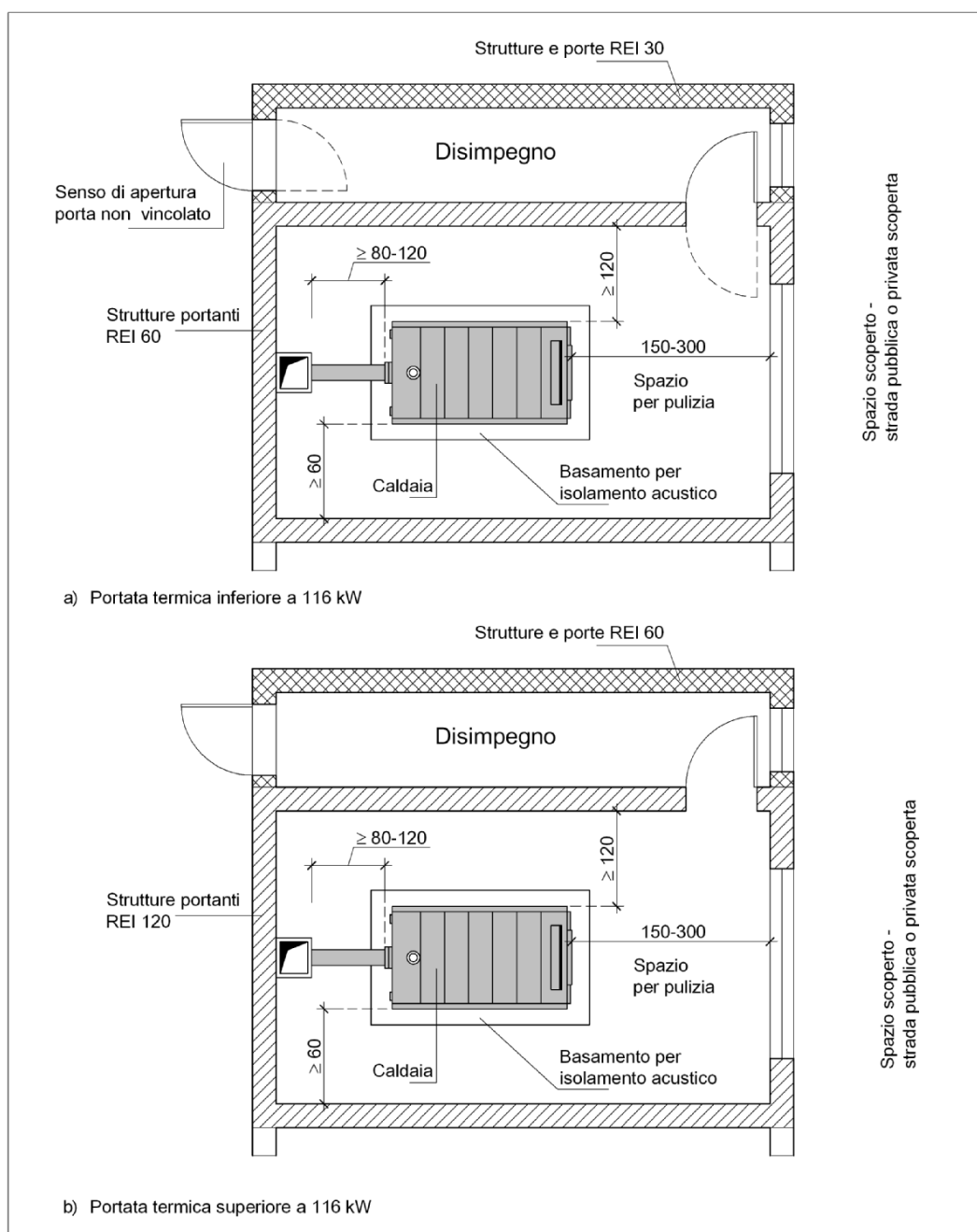
Figura 90.10 - Esempio di centrale termica alimentata a gas di rete con accesso da disimpegno con parete attestata su spazio esterno o da strada pubblica o privata scoperta. Caratteristiche costruttive e distanze minime consigliate per gli spazi attorno al generatore
