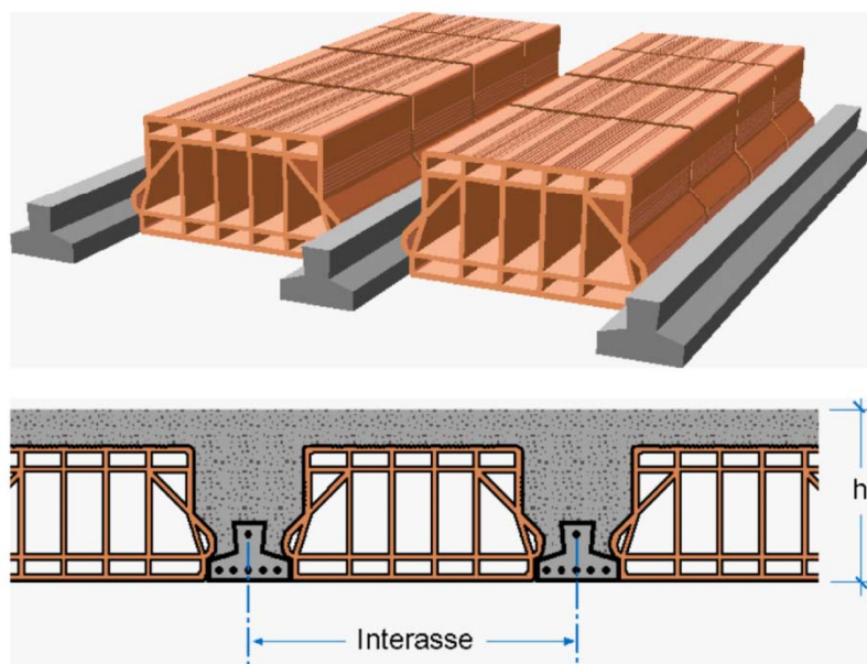
Figura 23.3 - Esempio di solaio in cemento armato a travetti in cemento armato e blocchi interposti 1
