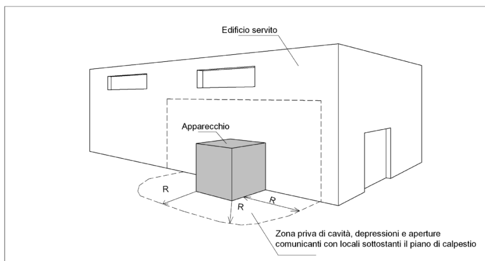
Figura 90.3 - Distanze da rispettare per l'installazione all'aperto degli apparecchi alimentati con gas a densità maggiore di 0,8
