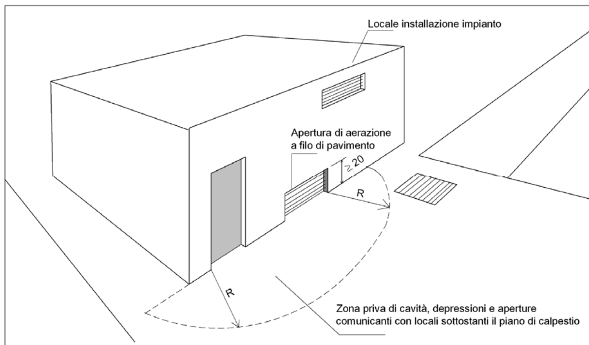
Figura 90.5 - Ulteriori prescrizioni per le aperture di aerazione del locale centrale termica fuori terra, alimentato a gas di rete con densità superiore a 0,8, come prescritto dal D.M. 12 aprile 1996
