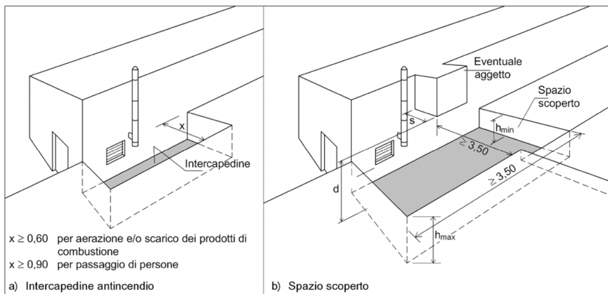
Figura 90.6 - Intercompartimento antincendio e spazio scoperto secondo il D.M. 30 novembre 1983
