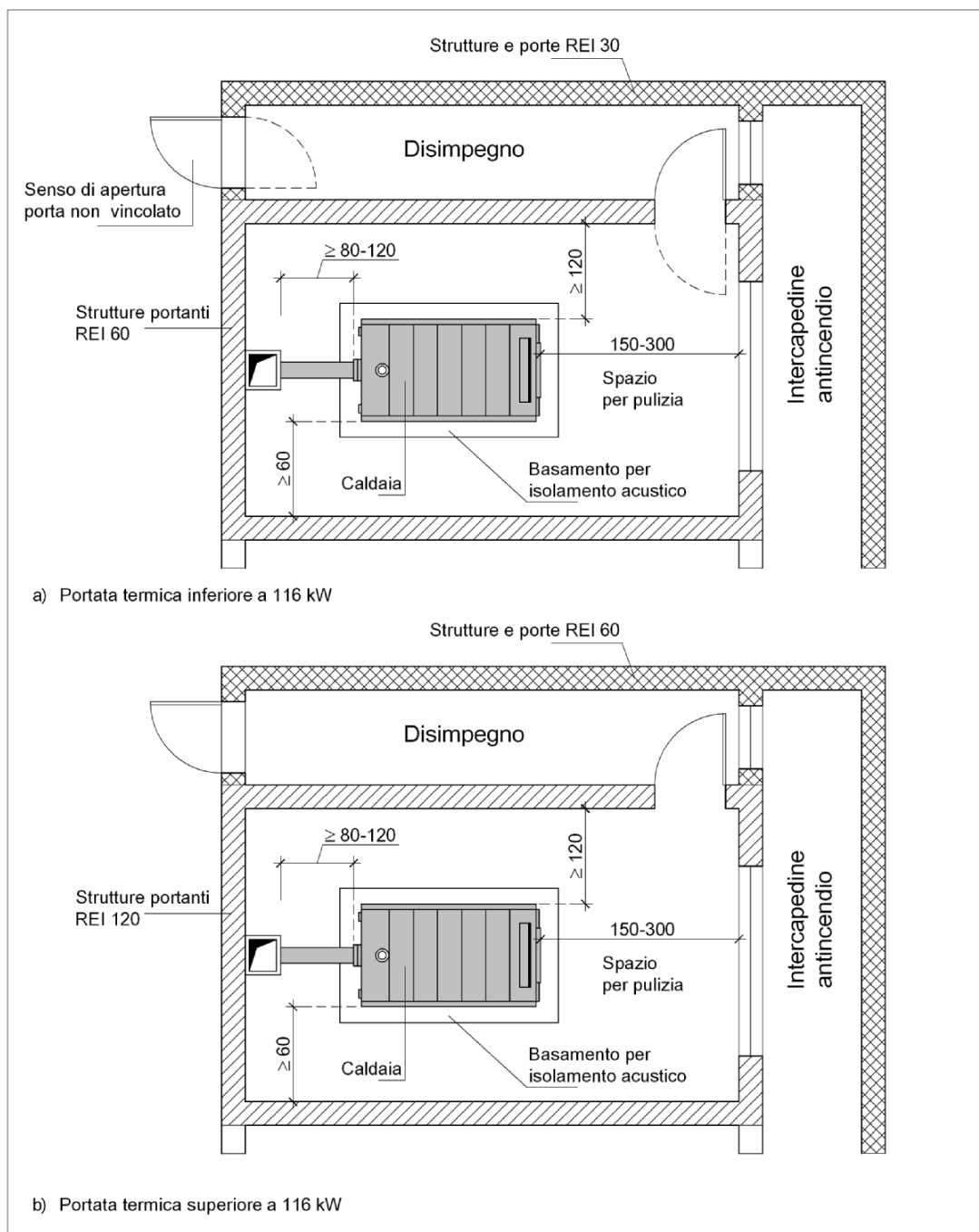
Figura 90.9 - Esempio di centrale termica alimentata a gas di rete con accesso da disimpegno con parete attestata su intercapedine antincendio. Caratteristiche costruttive e distanze minime consigliate per gli spazi attorno al generatore
