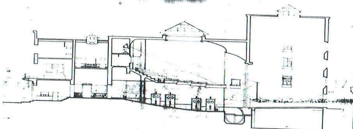
CINEMA-TEATRO-RIDOLA — SEZIONE LONGITUDINALE — RAPP. 1:50
