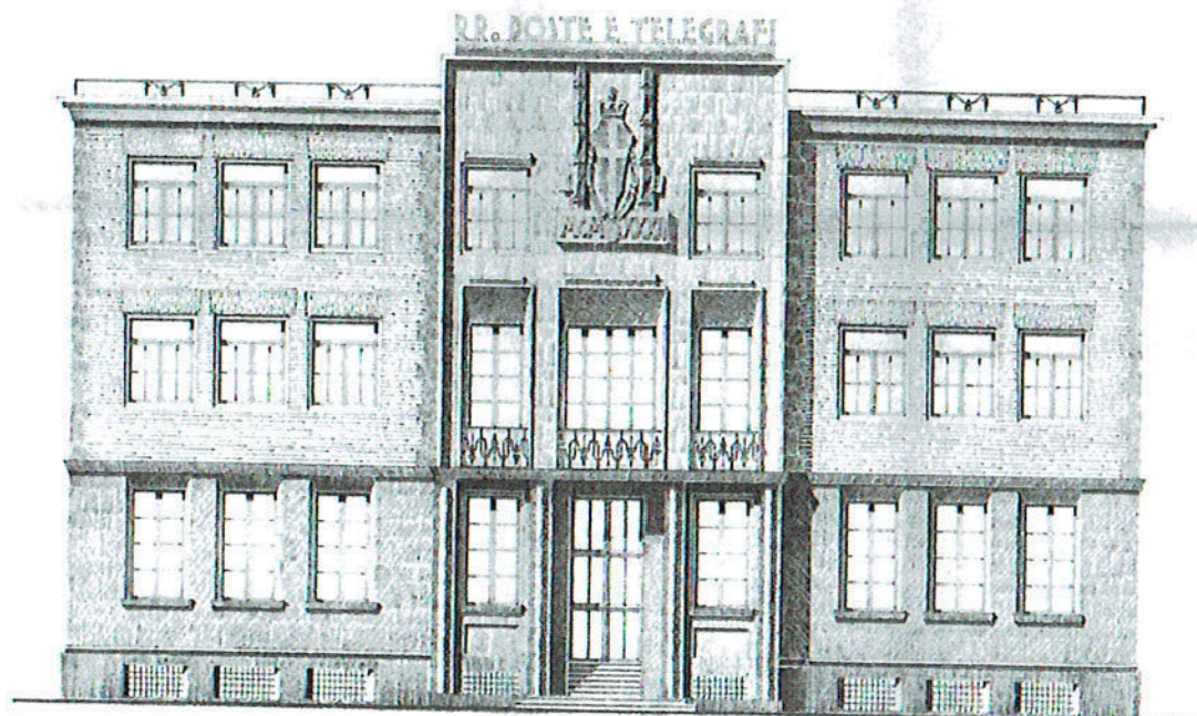
• PROSPETTO PRINCIPALE • RAPP. 1:50
